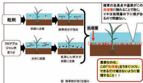
図2 除草剤が効く仕組み
